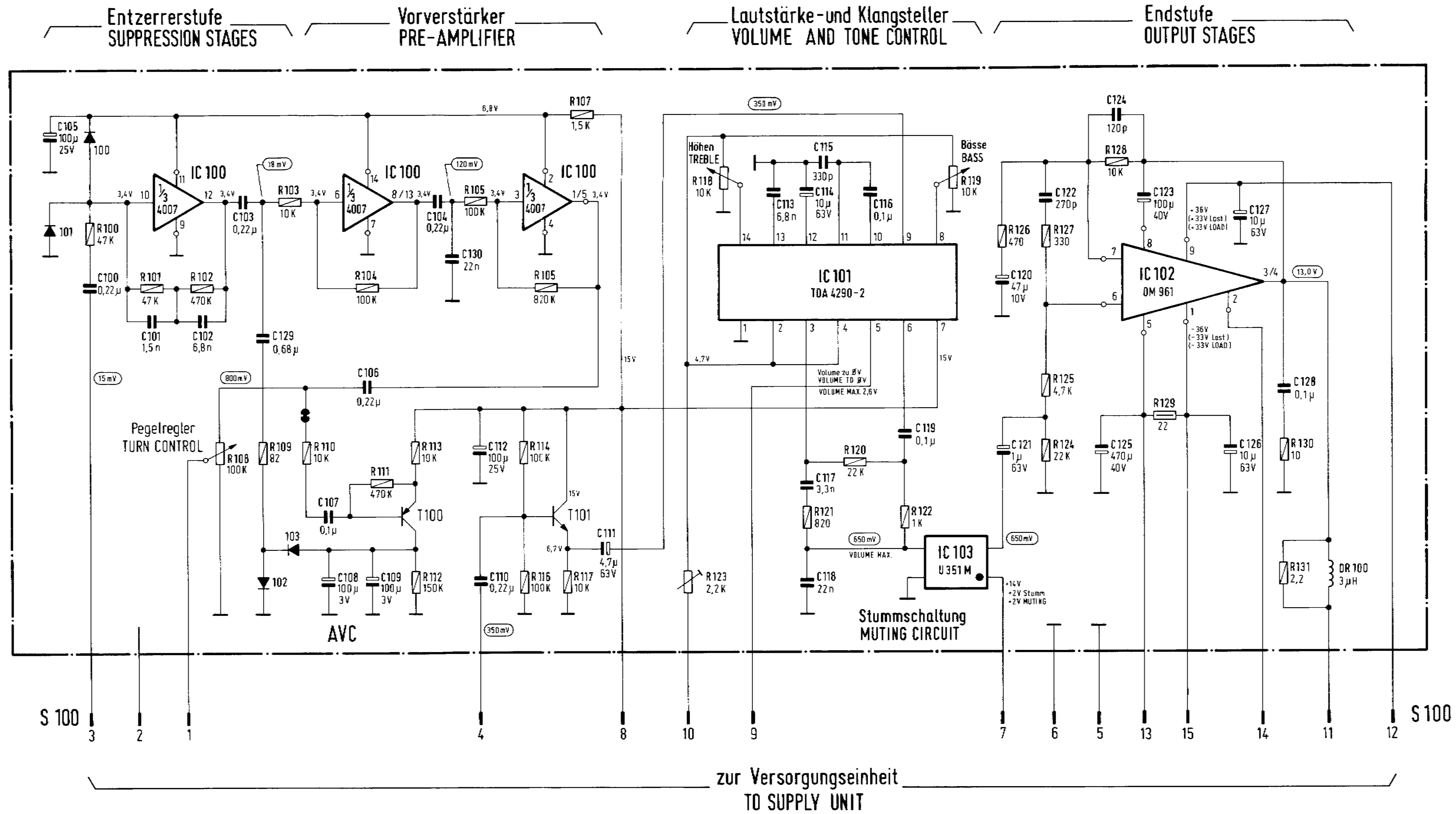
Schaltbild Verstärker WIRING DIAGRAM AMPLIFIER
